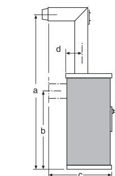
Maß a und c: mit Original-Winkelrohr dimension a and c: with original angle pipe Côtés a et c : avec conduit coudé d'origine Wymiary a i c : z oryginalną rurą pod kątem 90°
