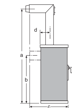
Maß a und c: mit Original-Winkelrohr dimension a and c: with original angle pipe Côtés a et c : avec conduit coudé d'origine Wymiary a i c : z oryginalną rurą pod kątem 90°
